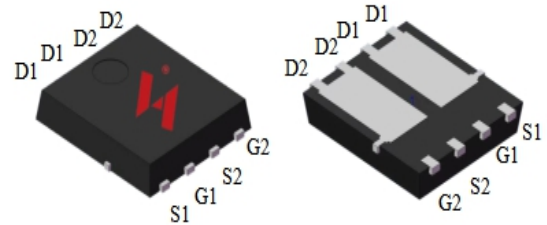
PDFN8L(5x6)
