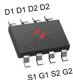
SOP8L
