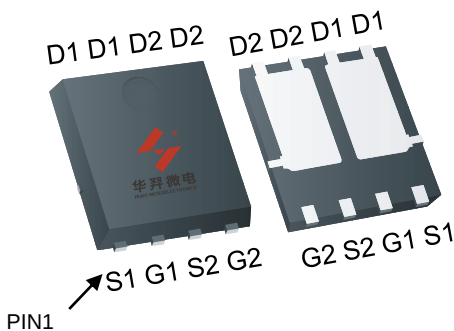
PDFN8L(5x6)
