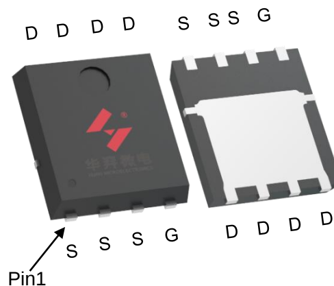
PDFN8L(5x6)
