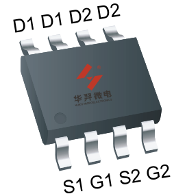
SOP8L
