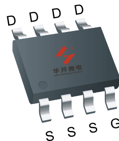
SOP8L
