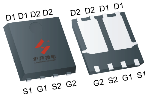
PDFN8L(5×6)
