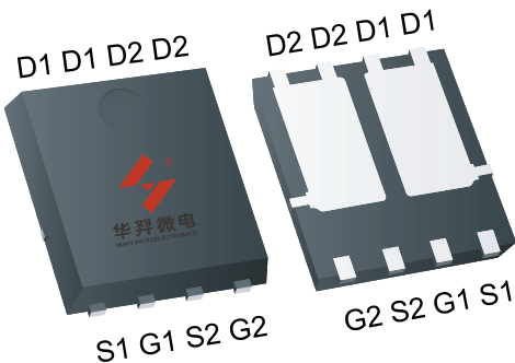
PDFN8L(5x6)
