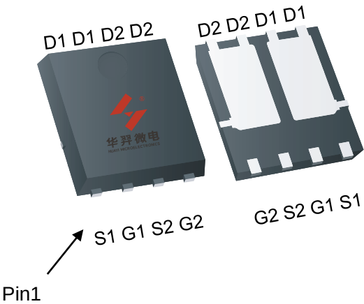
PDFN8L(5x6)
