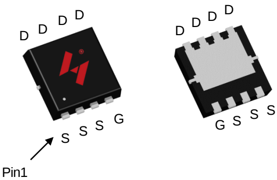
PDFN8L (3.3*3.3)
