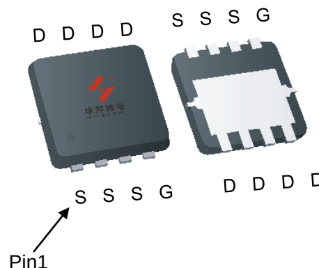
PDFN8L(3.3x3.3)
